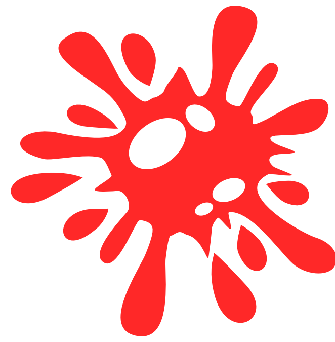
ROUGE
