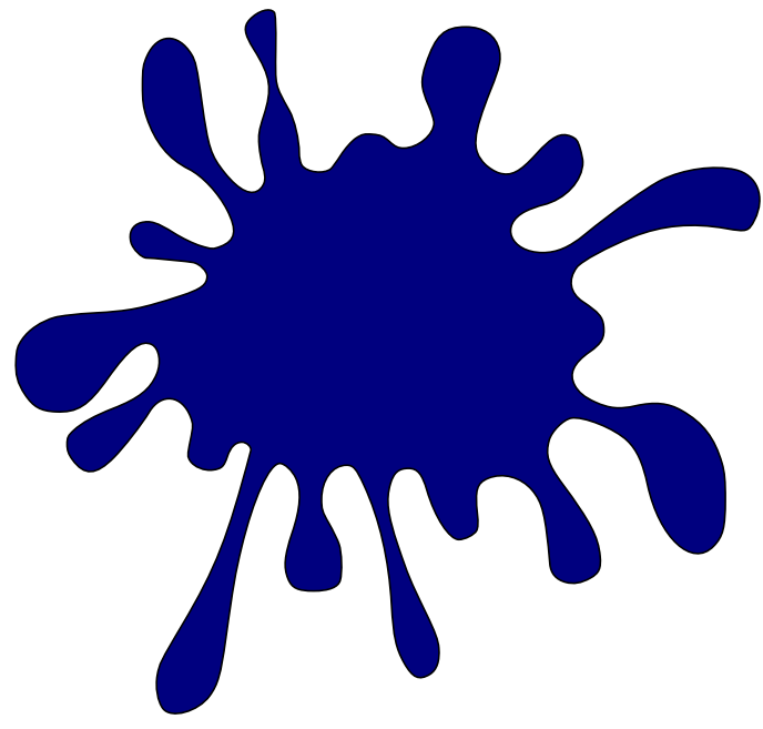
BLEU
